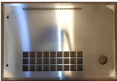
PN: 14831 Door Generator, 5.5 Onan, Clamshell
